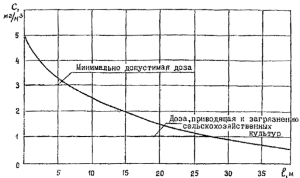
Рис. 3 Загазованность придорожной территории на автомобильной дороге III категории ( N=3000 авт/сут) выбросами автотранспорта (окись углерода)
