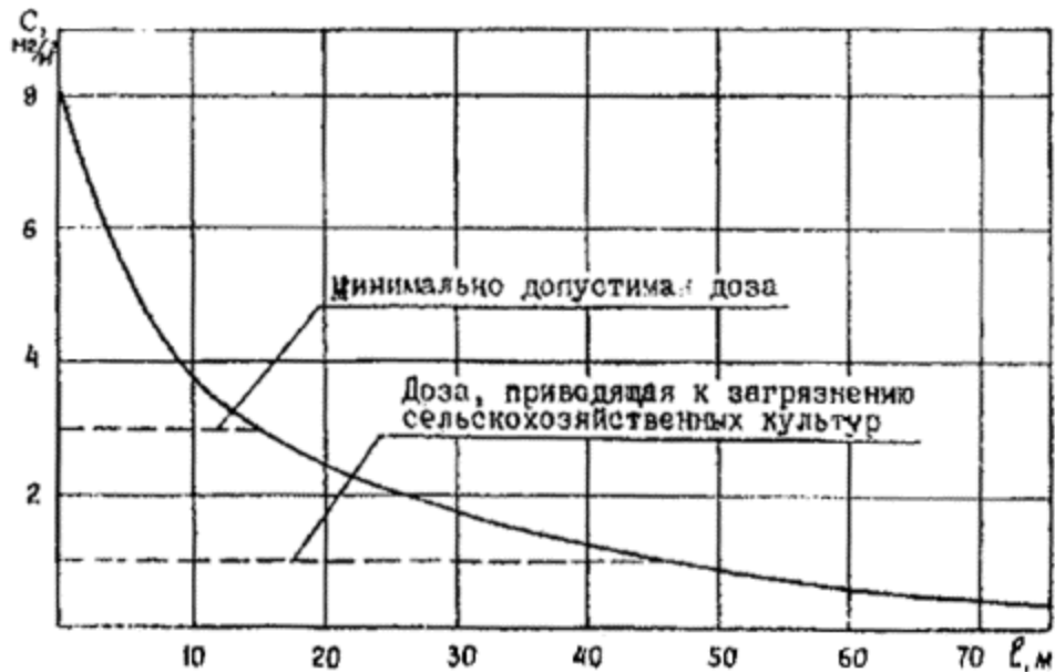
Рис. 2 Загазованность придорожной территории на автомобильной дороге II категории ( N=5000 авт/сут), выбросами автотранспорта (окись углерода)
