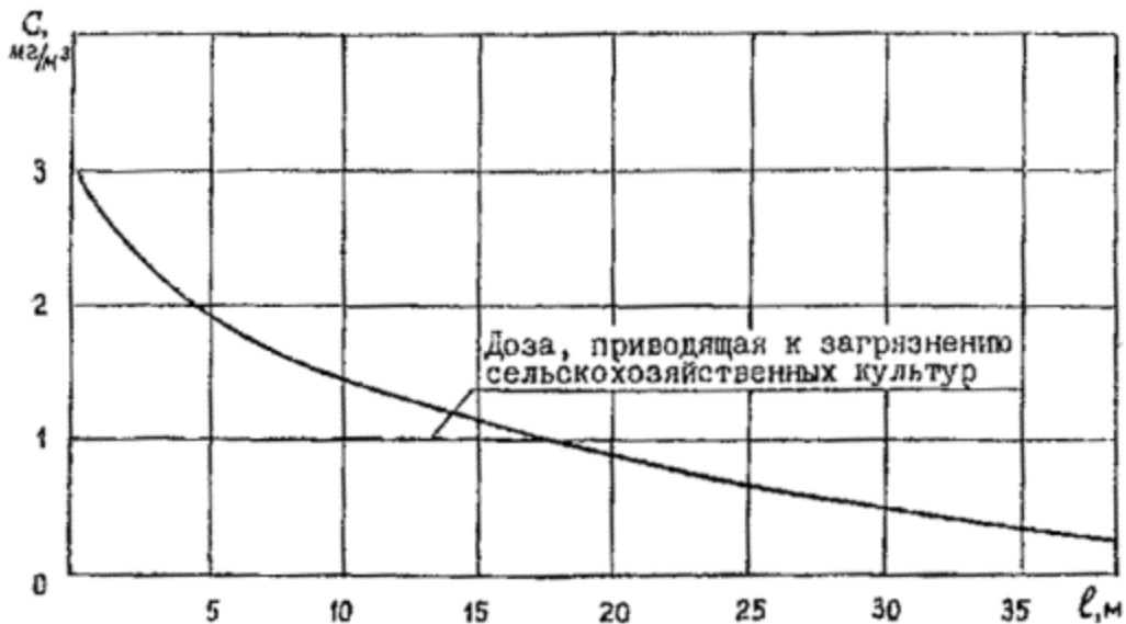
Рис. 4 Загазованность придорожной территории на автомобильной дороге IV категории ( N=1000 авт./сут.) выбросами автотранспорта (окись углерода)
