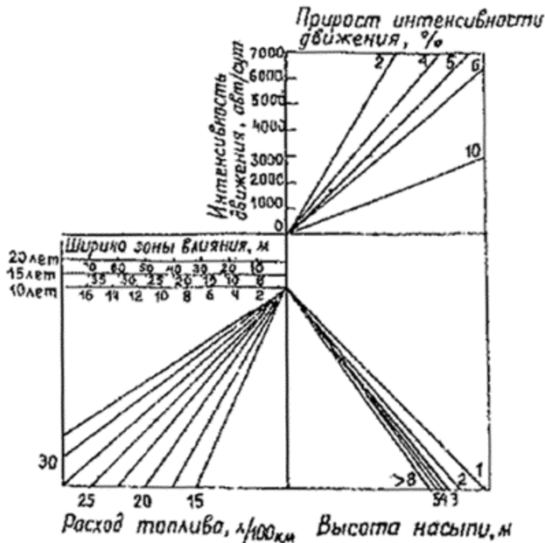
Рис. 8 Номограмма для определения ширины зоны влияния загрязнения придорожной полосы выбросами автомобильного транспорта тяжелыми металлами в зависимости от высоты насыпи, прироста интенсивности движения, расхода топлива ( P ).
